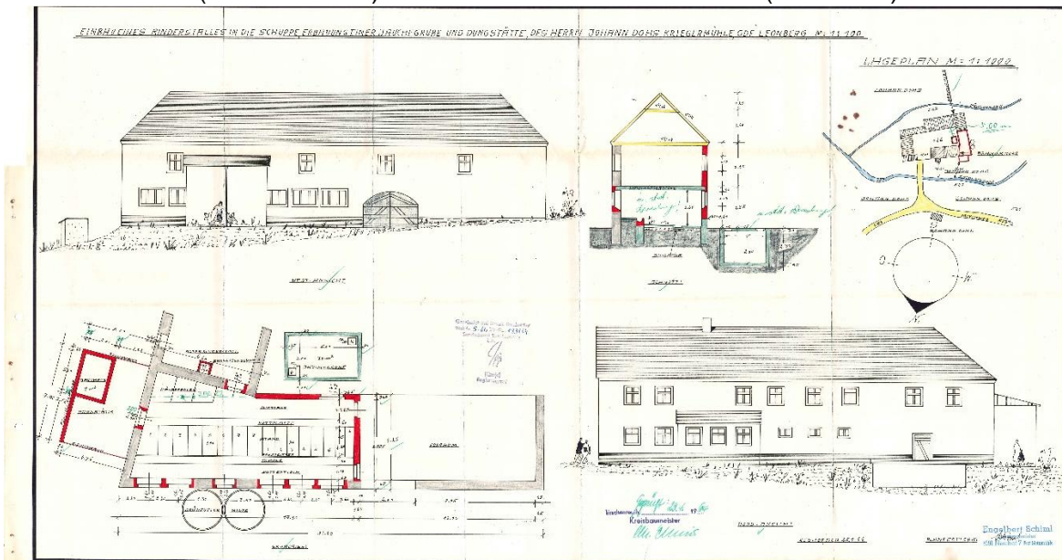
Plan mit Grundriss Stall
